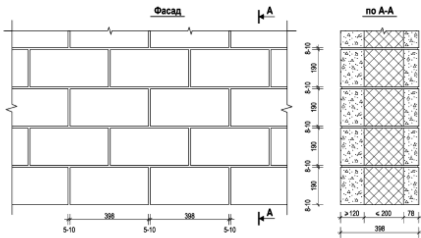
Рис.1. Кладка наружных стен однопорядной системы перевязки из трехслойных блоков
