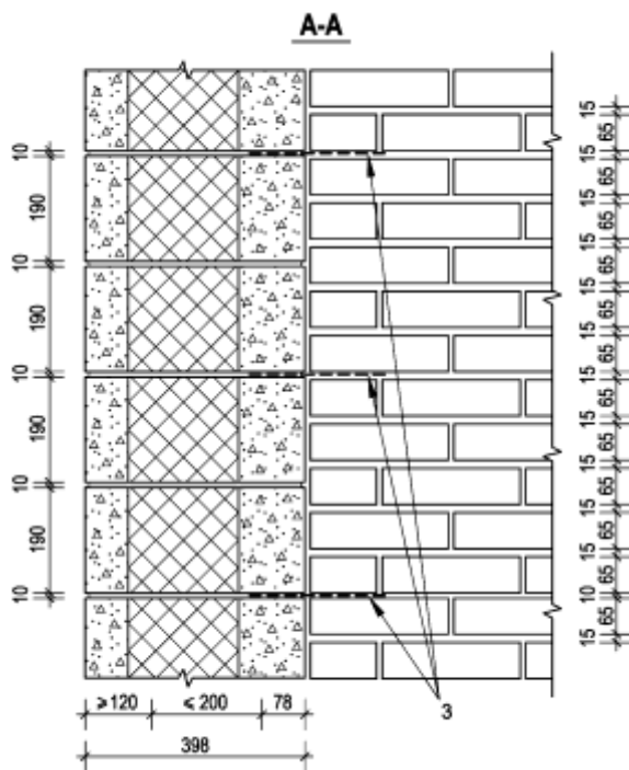
Рис.12. Узел сопряжения наружных стен и перегородок
