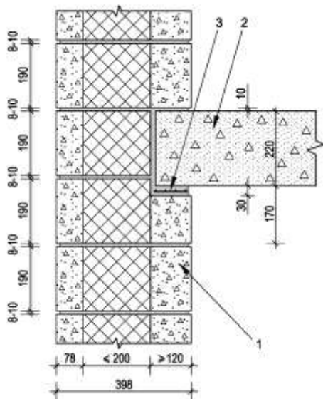
Рис.3. Узлы опирания плиты перекрытия на несущие наружные стены из трехслойных стеновых блоков а) опирание плиты перекрытия на армокирпичный пояс б) опирание плиты перекрытия на трехслойный блок
