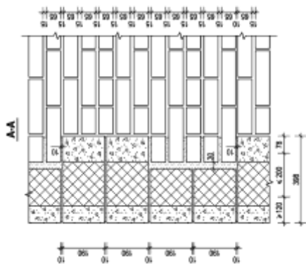
Рис. 11. Узлы сопряжения наружных и внутренних стен
