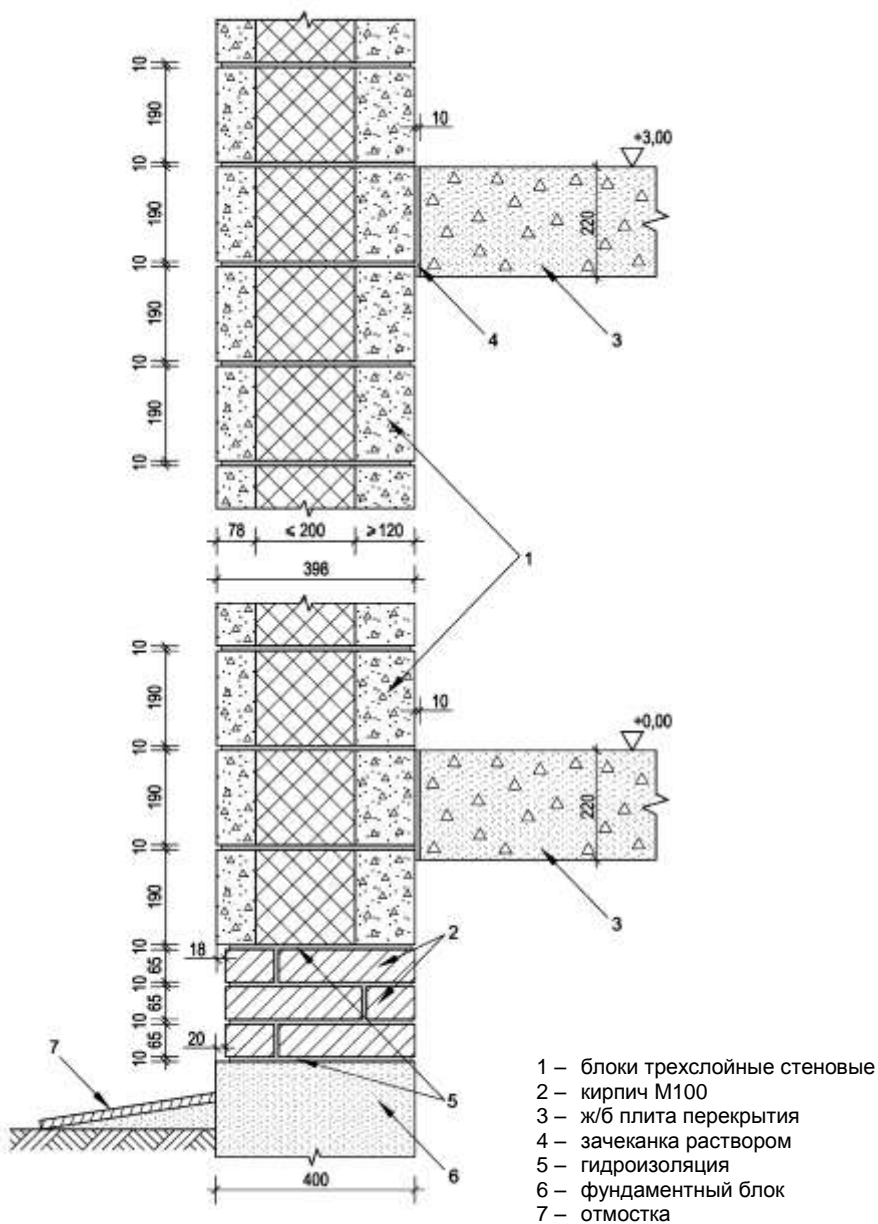
Рис.5. Схема кладки самонесущих наружных стен из трехслойных стеновых блоков
