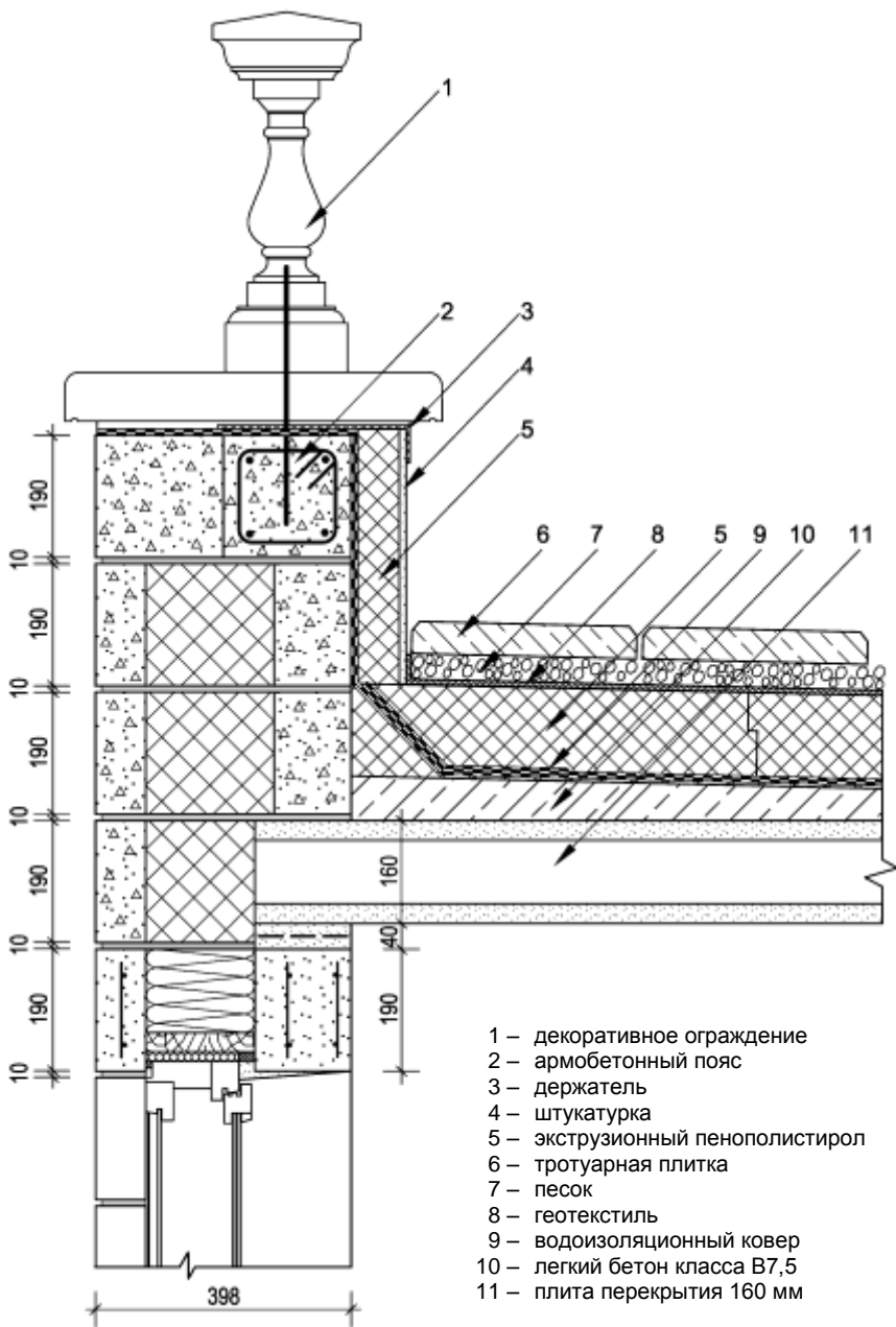
Рис.10. Сопряжение наружной стены из трехслойных блоков с плоской инверсионной кровлей
